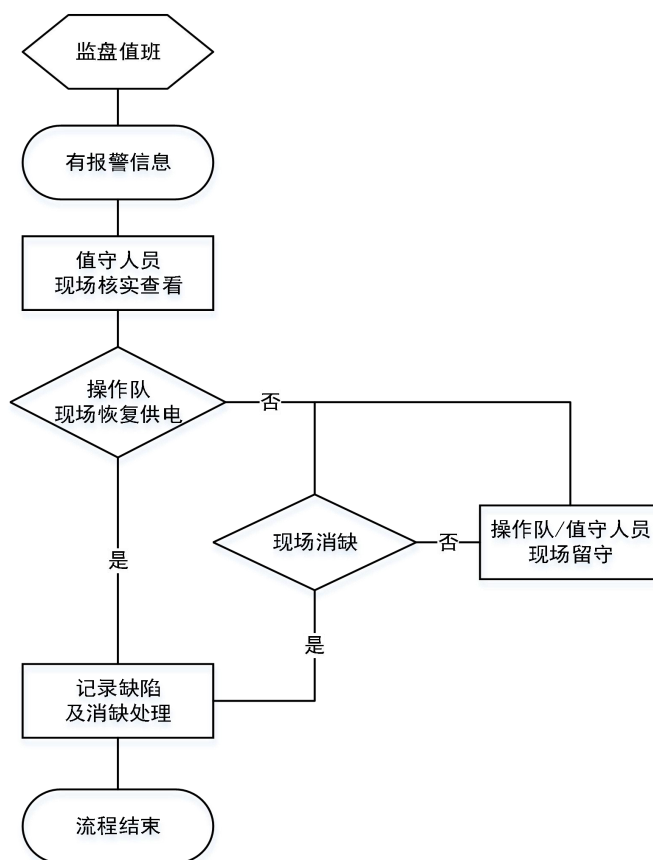
图4 报警及故障抢修状态下的运维流程图
