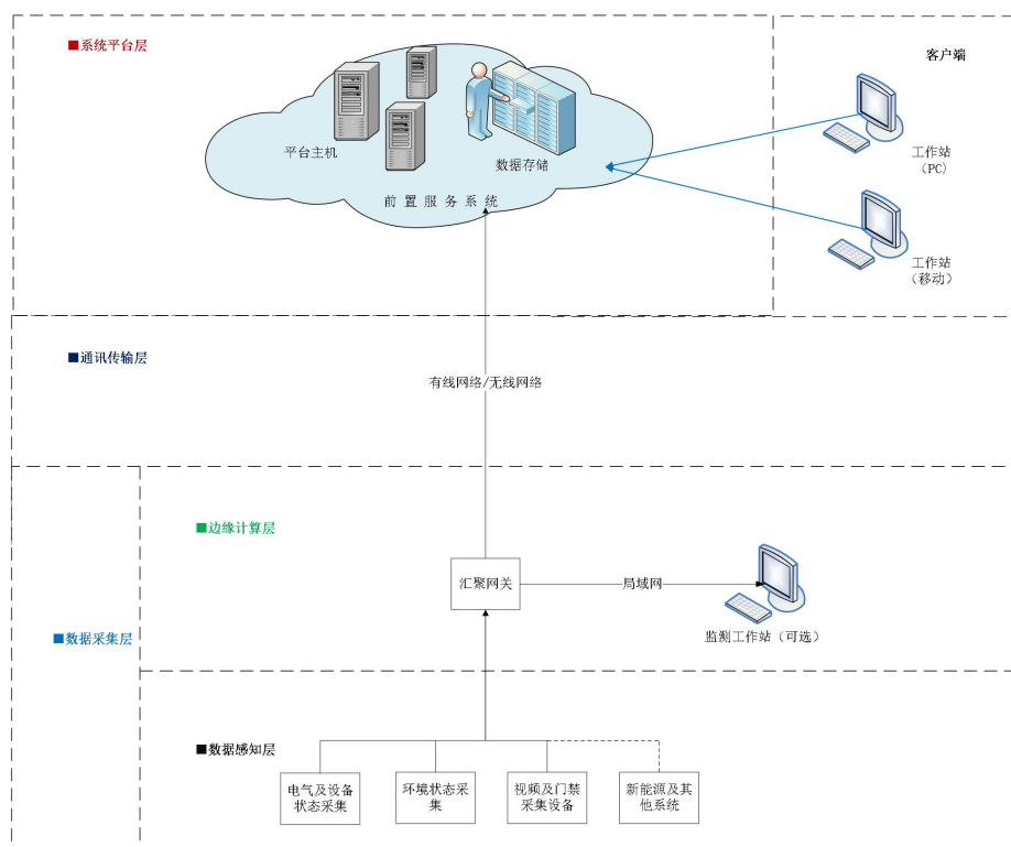
图 1 系统架构
